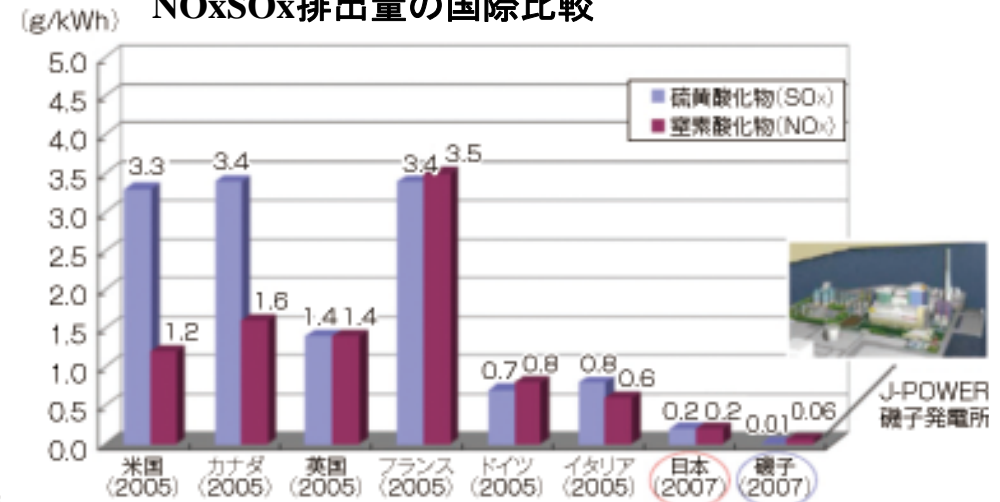
石炭火力発電からの電力1kWhあたりのNO x SO x 排出量の国際比較
