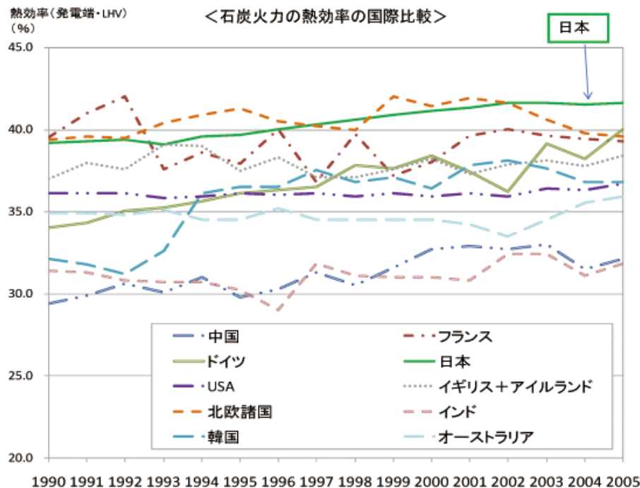
石炭火力発電所の熱効率の各国比較
