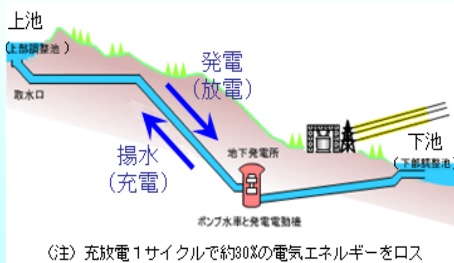
揚水式水力発電
