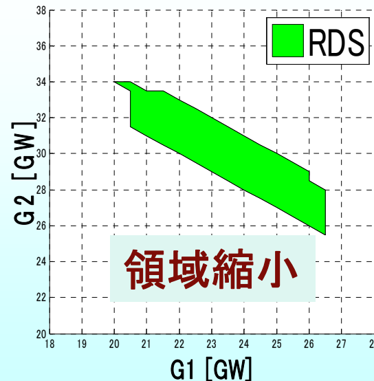
PV予測誤差:20%
