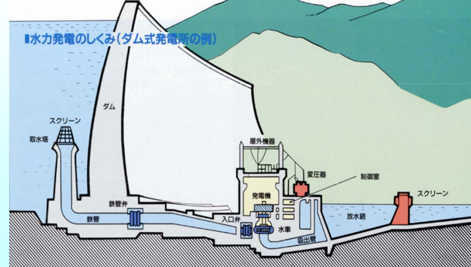
ダム式水力発電
